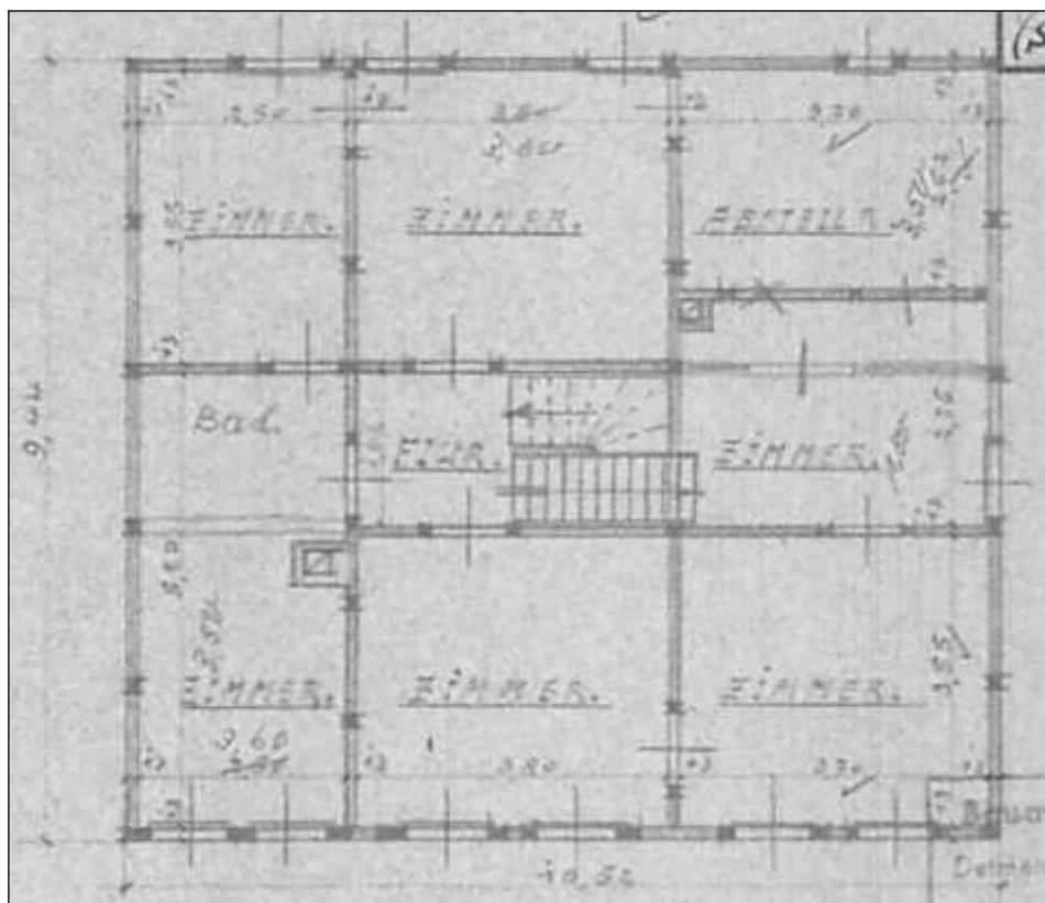
- Obergeschoss -
